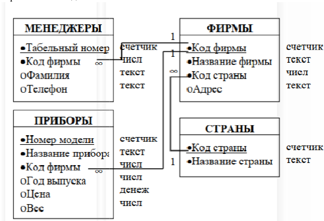
Рис. 13. Реляционная модель БД «Приборы».
